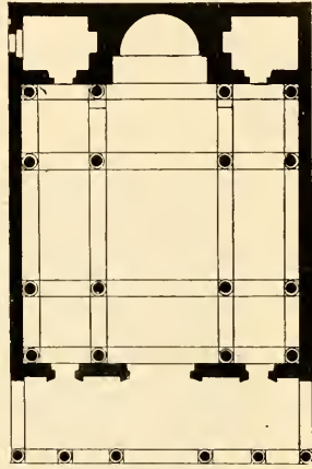
Fig. 2 — Pianta della chiesa di Mousmich in Siria (sec. II e sec. III)
